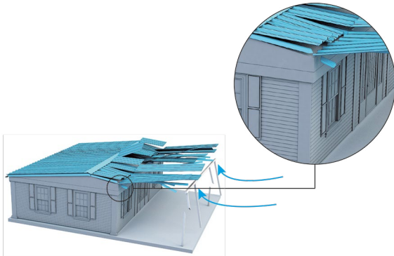
Figure 10 : Cas d'un auvent solidaire
