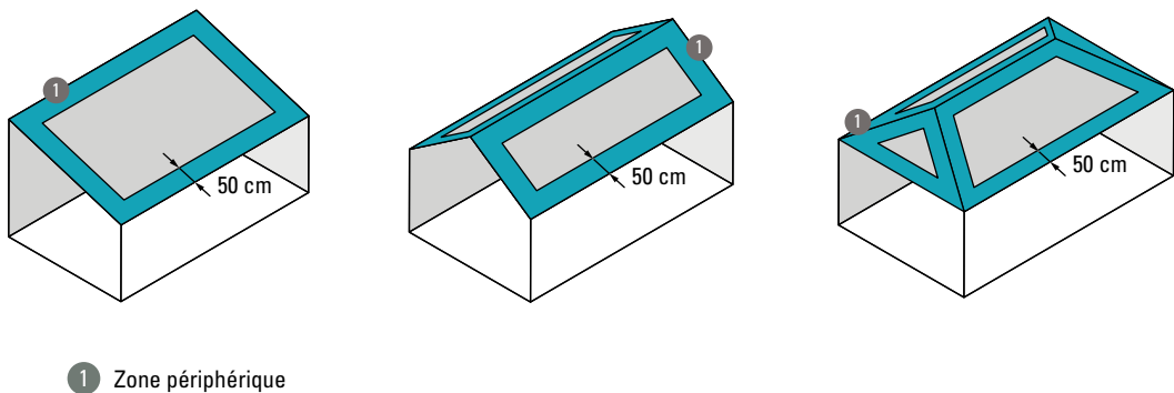
Figure 19 : Zone périphérique pour une toiture à 1, 2 et 4 versants
