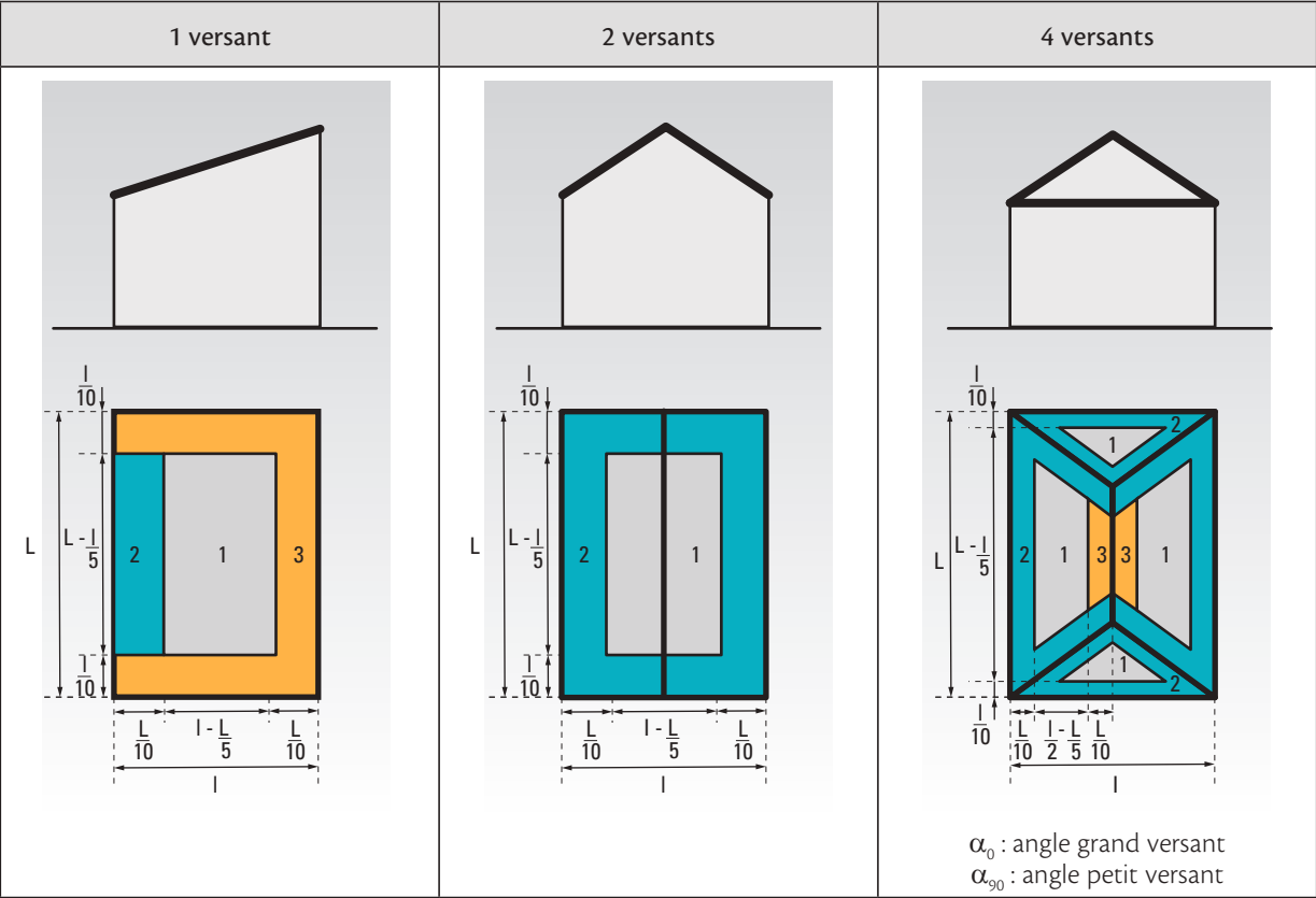
Figure 68 : Définition simplifiée des zones de toiture selon le nombre de versants
