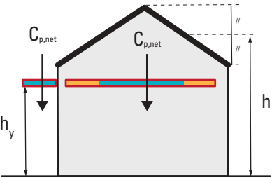
Figure 115 : Rapport h_1/h
