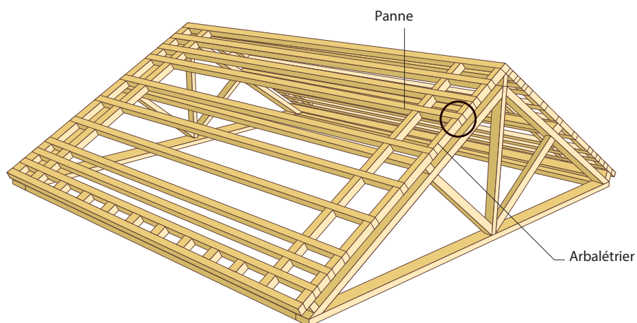
Figure 34 : Exemple de fixation des pannes sur l'arbalétrier
