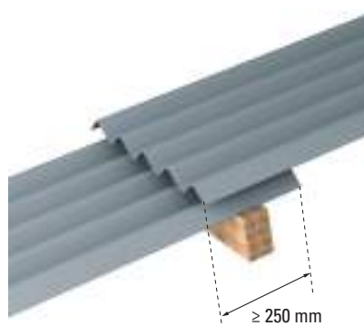
Figure 61 : Recouvrement minimum pour une tôle ondulée
