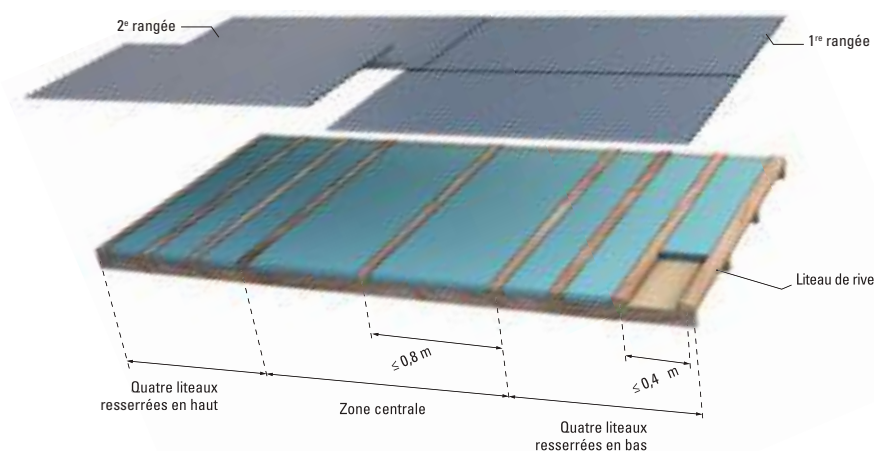
Figure 59 : Exemples de calepinage de deux rangées de plaques 8
