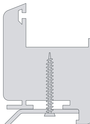
Figure 144 : Exemple de liaison patte/menuiserie
