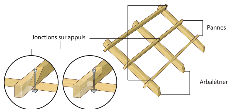
Figure 38 : Exemple de jonction éventuelle des pannes sur appuis à réaliser
