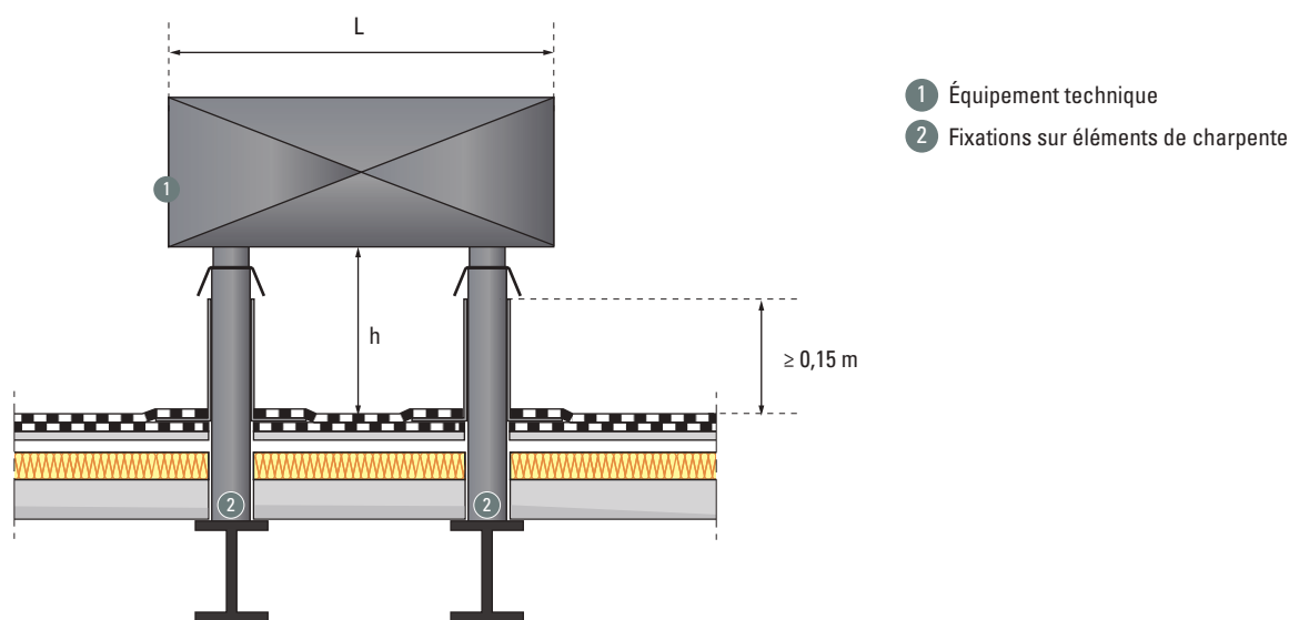
Figure 159 : Hauteur libre minimale
