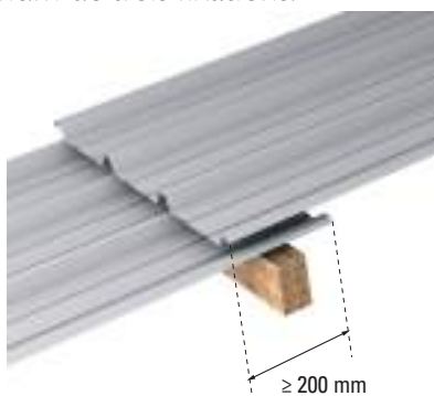
Figure 60 : Recouvrement minimum pour une tôle nervurée
