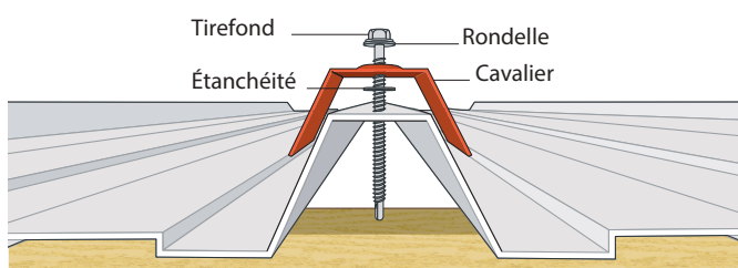
Figure 73 : Vue éclatée
