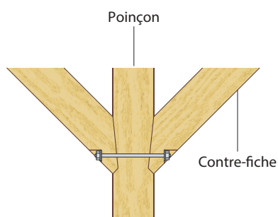
Figure 30 : Exemple d'assemblage contrefiche - poinçon par un boulon
