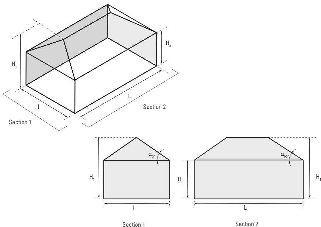
Figure 48 : Exemple de configuration avec la charpente à 4 versants
