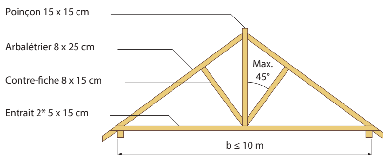
Figure 13 : Exemple de composants d'une ferme
