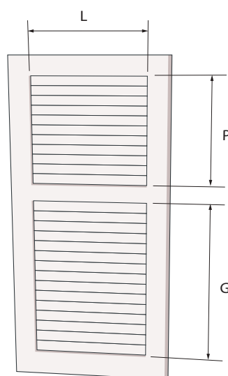
Figure 133 : Volet traditionnel ventilé (dit « à persienne »)
