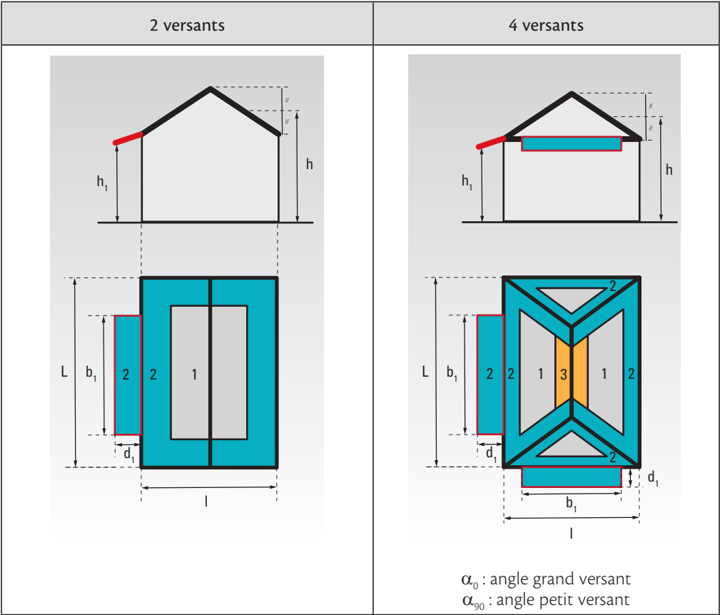
Figure 111 : Définition des zones de toiture selon le nombre de versants
