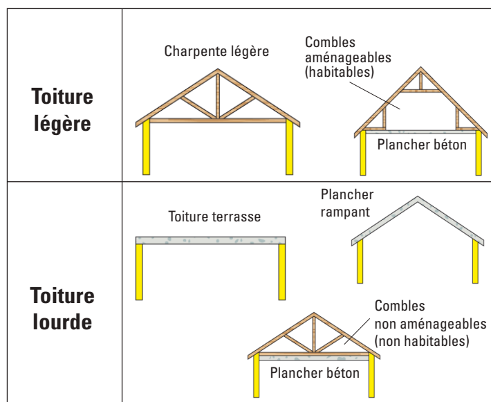
Figure 1 : Illustration des types de toitures 5
