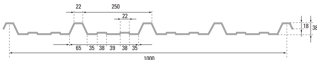
Figure 57 : Exemples de dimensions standards de tôle nervurée
