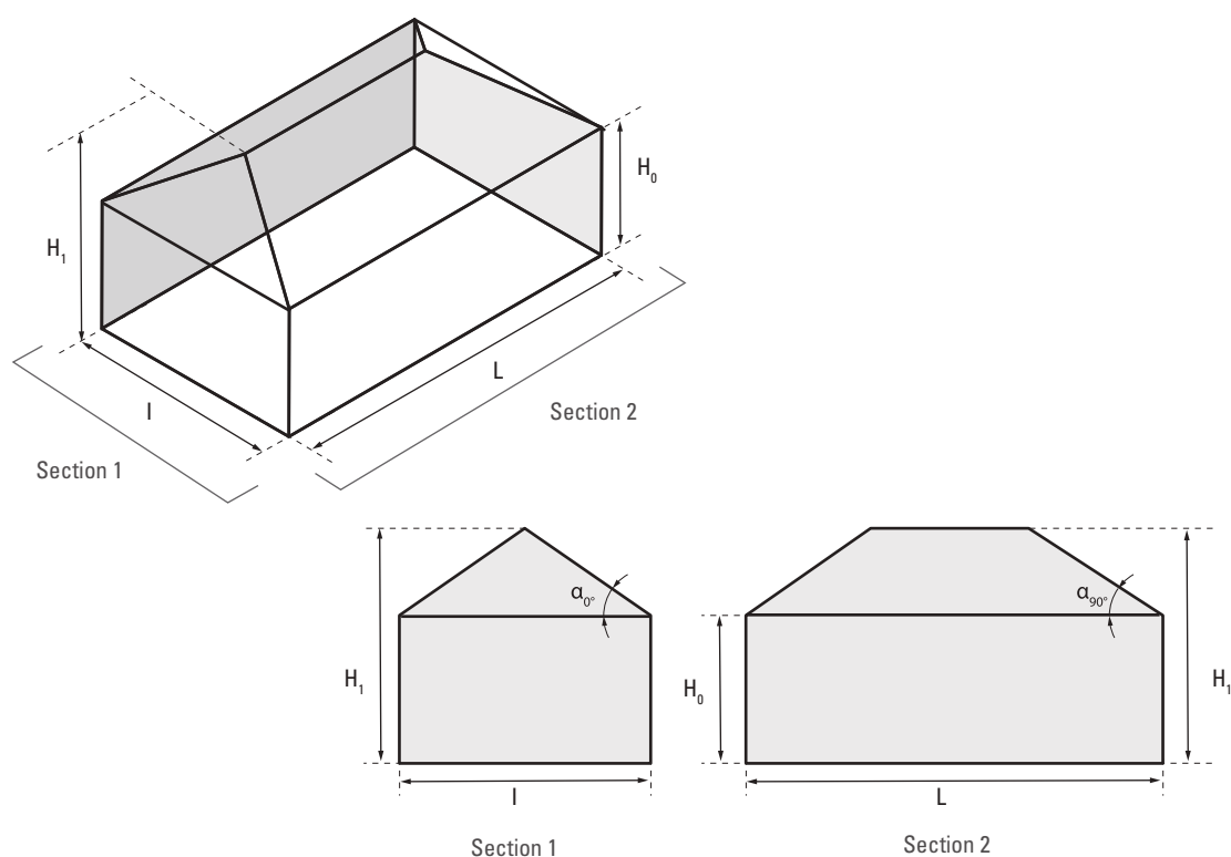
Figure 24 : Exemple de configuration avec la charpente à 4 versants
