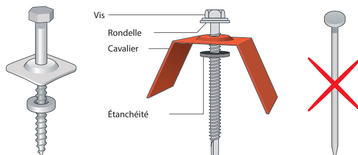
Figure 71 : Exemples de fixations
