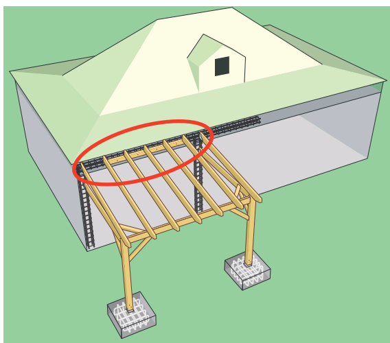
Figure 107 : Exemple de contreventement par bracon
