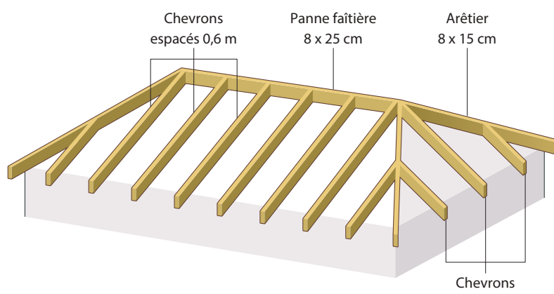
Figure 14 : Exemple d'une charpente à 4 versants
