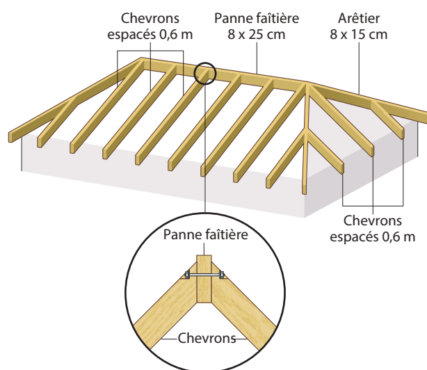
Figure 39 : Exemple de fixation des chevrons sur la panne faîtière par un boulon
