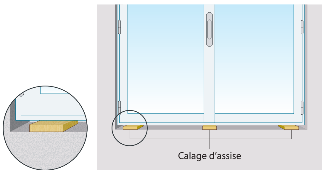
Figure 148 : Exemple de calage
