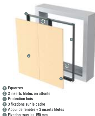
Figure 126 : Exemple d'un principe de protection provisoire
