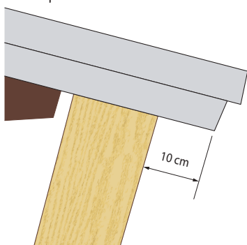
Figure 62 : Débord maximal de la couverture en rive basse sans renfort
