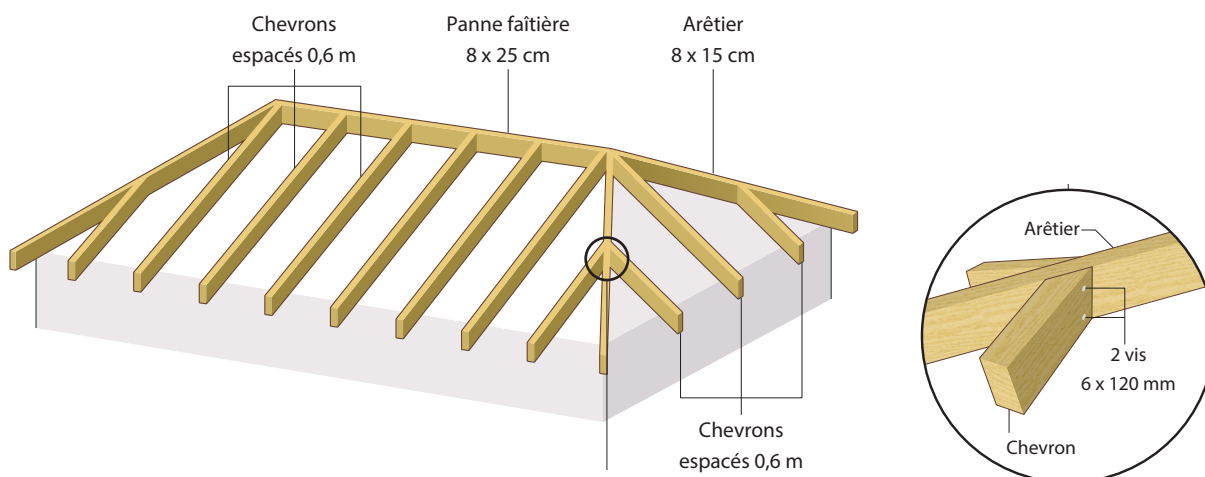
Figure 40 : Exemple de fixation des chevrons sur la panne faîtière par un boulon
