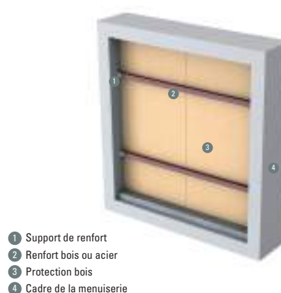
Figure 122 : Renfort de protection
