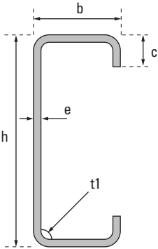
Figure 51 : Exemple de configurations étudiées des pannes en profilés métalliques minces de forme en C
