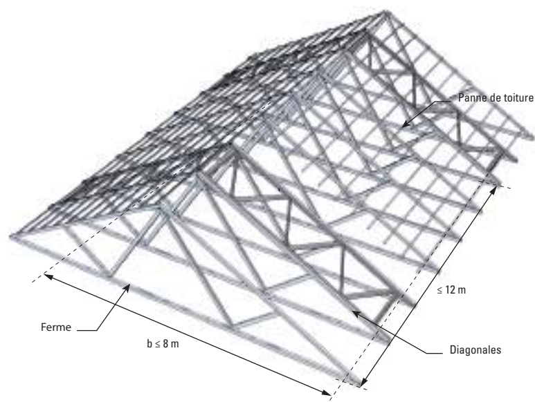
Figure 45 : Exemple de triangulation en croix de Saint-André
