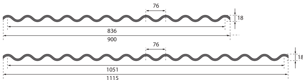
Figure 56 : Exemples de dimensions standards de tôle ondulée
