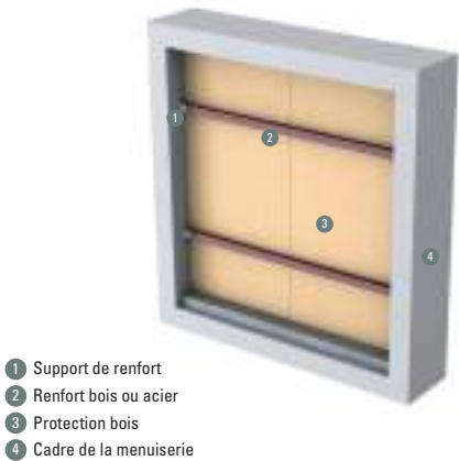
Figure 140 : Exemple de protection provisoire aux chocs renforcée
