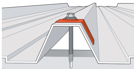
Figure 72 : Vis dans une panne métallique
