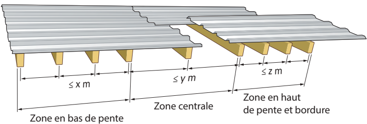
Figure 114 : Exemple d'une couverture d'auvent à un versant – définition de trois zones
