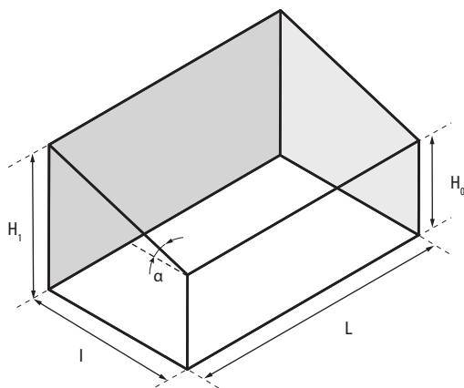
Figure 46 : Exemple de configuration avec la charpente à 1 versant
