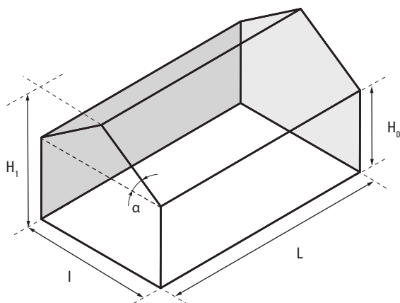
Figure 47 : Exemple de configuration avec la charpente à 2 versants
