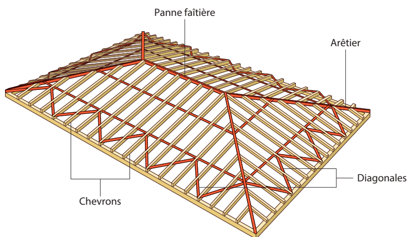
Figure 19 : Exemple de diagonales mises en œuvre pour une charpente à 4 versants
