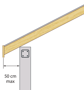
Figure 63 : Débord maximal de la couverture en rive basse avec prolongement de la charpente
