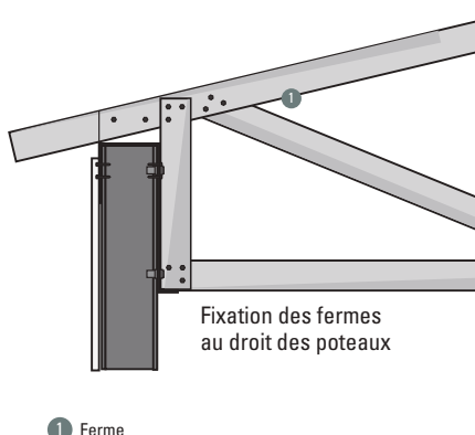
Figure 53 : Exemple de fixation des fermes au droit des poteaux
