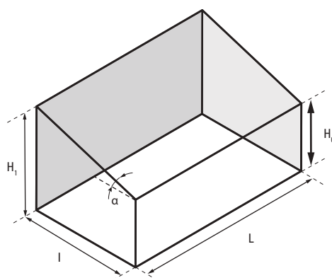
Figure 22 : Exemple de configuration avec la charpente à 1 versant
