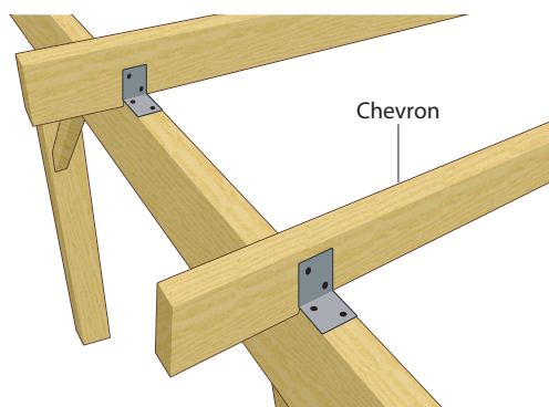
Figure 118 : Exemple de sabot à ailes extérieures inox
