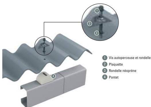
Figure 74 : Fixation d'une tôle ondulée avec pontet
