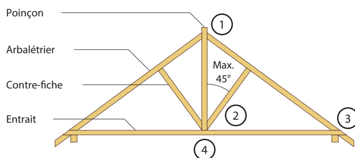
Figure 28 : Exemple d'assemblages des éléments de la ferme
