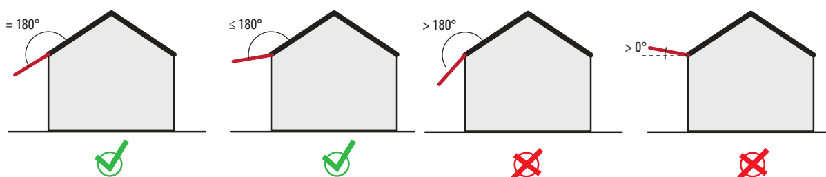
Figure 112 : Cas couverts par le calcul
