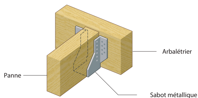
Figure 35 : Exemple de fixation des pannes sur l'arbalétrier par des sabots métalliques
