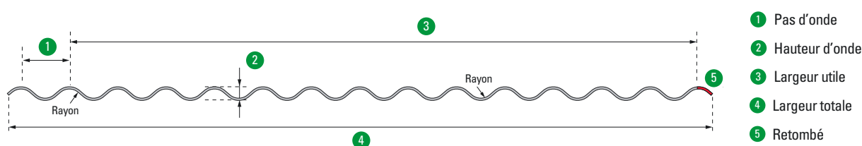
Figure 55 : Plaques ondulées – dénominations et paramètres
