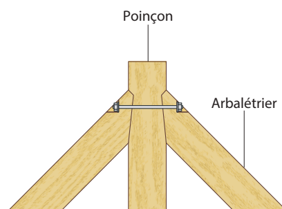
Figure 29 : Exemple d'assemblage poinçon-arbalétrier par un boulon
