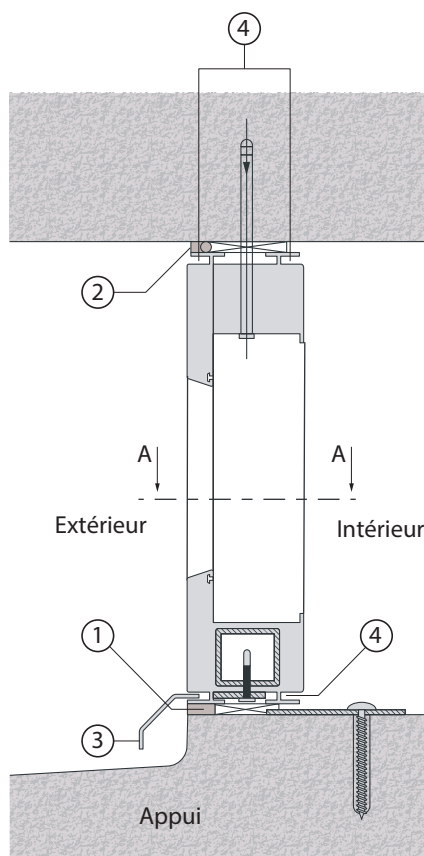
Figure 150 : Mise en œuvre en tableau
