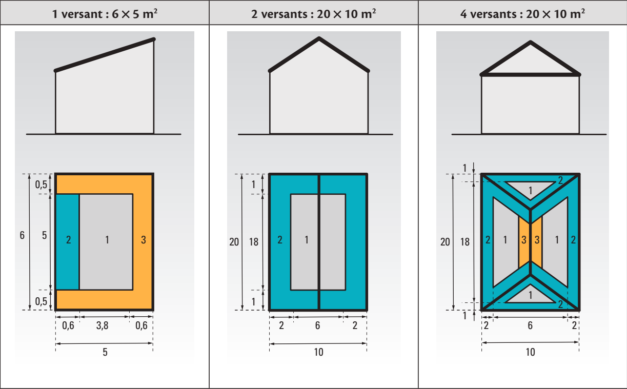
Figure 26 : Exemples de dimensions des zones de toiture selon le nombre de versants
