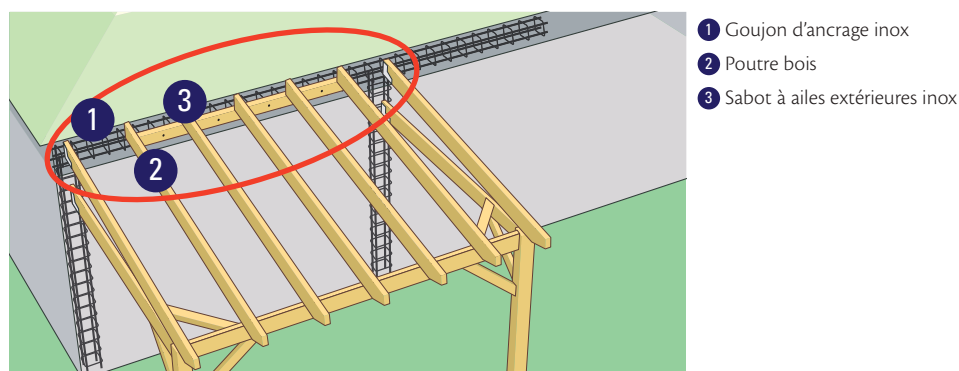
Figure 119 : Exemple de fixation à la façade du bâtiment
