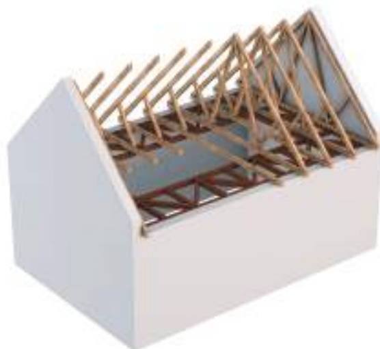
Figure 20 : Exemple de contreventement d'une charpente à 2 versants par poutres au vent horizontales dans le plan des entrails
