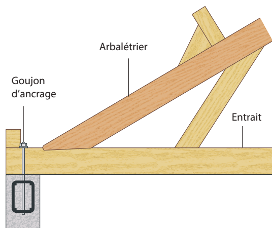
Figure 41 : Exemple d'ancrage de la charpente dans le béton par goujon d'ancrage
