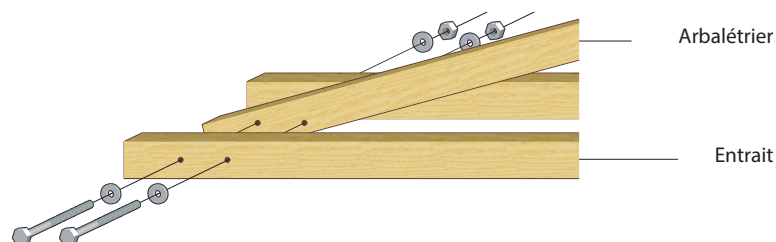
Figure 32 : Exemple d'assemblage entrain moisé - arbalétrier par 2 boulons
