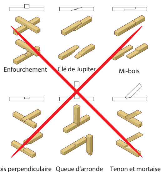
Figure 27 : Exemple d'assemblages de charpentiers nécessitant des dispositifs assurant leur maintien en position, même avec une inversion des efforts
