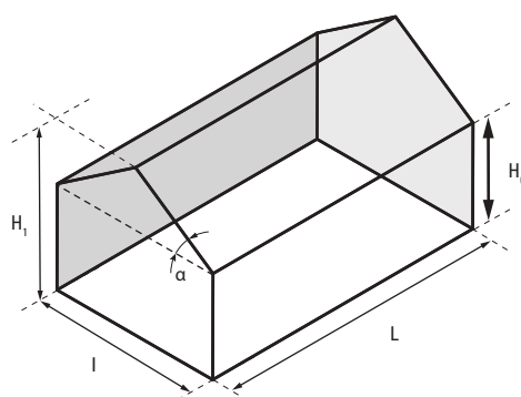
Figure 23 : Exemple de configuration avec la charpente à 2 versants
