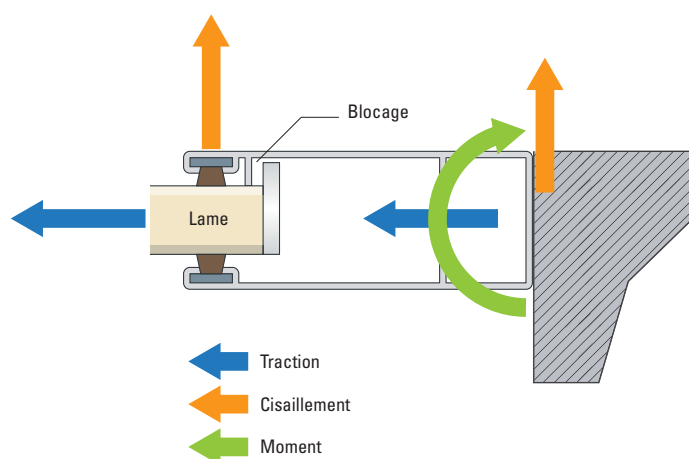
Figure 137 : Risque de rupture localisé du support par poussée au vide et/ou arrachement de la fixation
