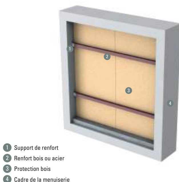
Figure 129 : Exemple de protection provisoire renforcée
