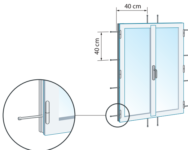
Figure 147 : Exemple de fixation par « vis à béton »
