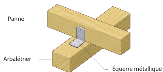
Figure 36 : Exemple de fixation des pannes sur l'arbalétrier par des équerres métalliques
