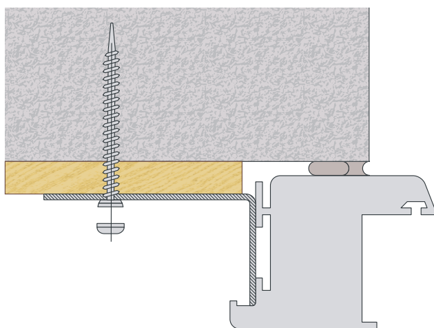
Figure 143 : Exemple de fixation par patte
