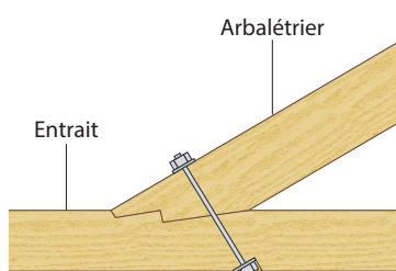
Figure 31 : Exemple d'assemblage entrain - arbalétrier par un boulon
