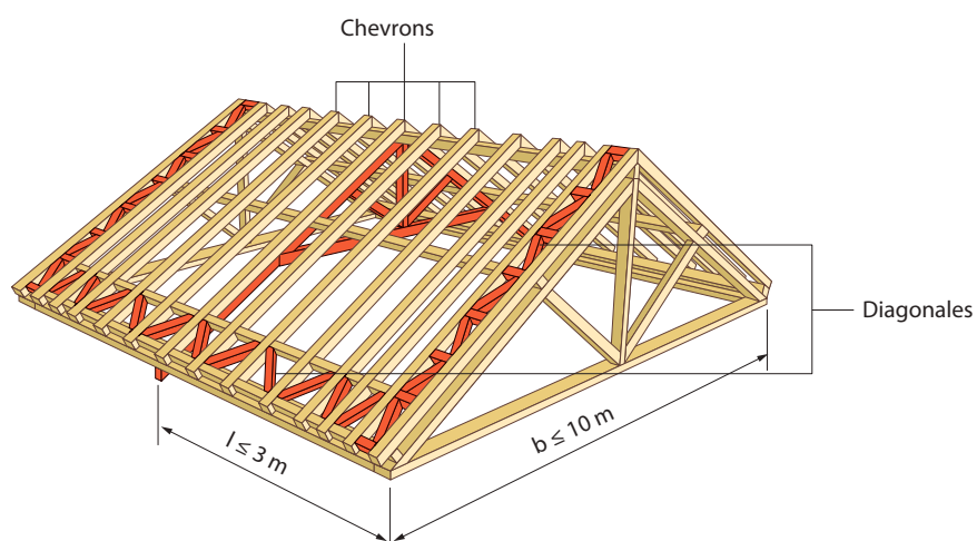
Figure 17 : Exemple de diagonales mises en œuvre entre chevrons
