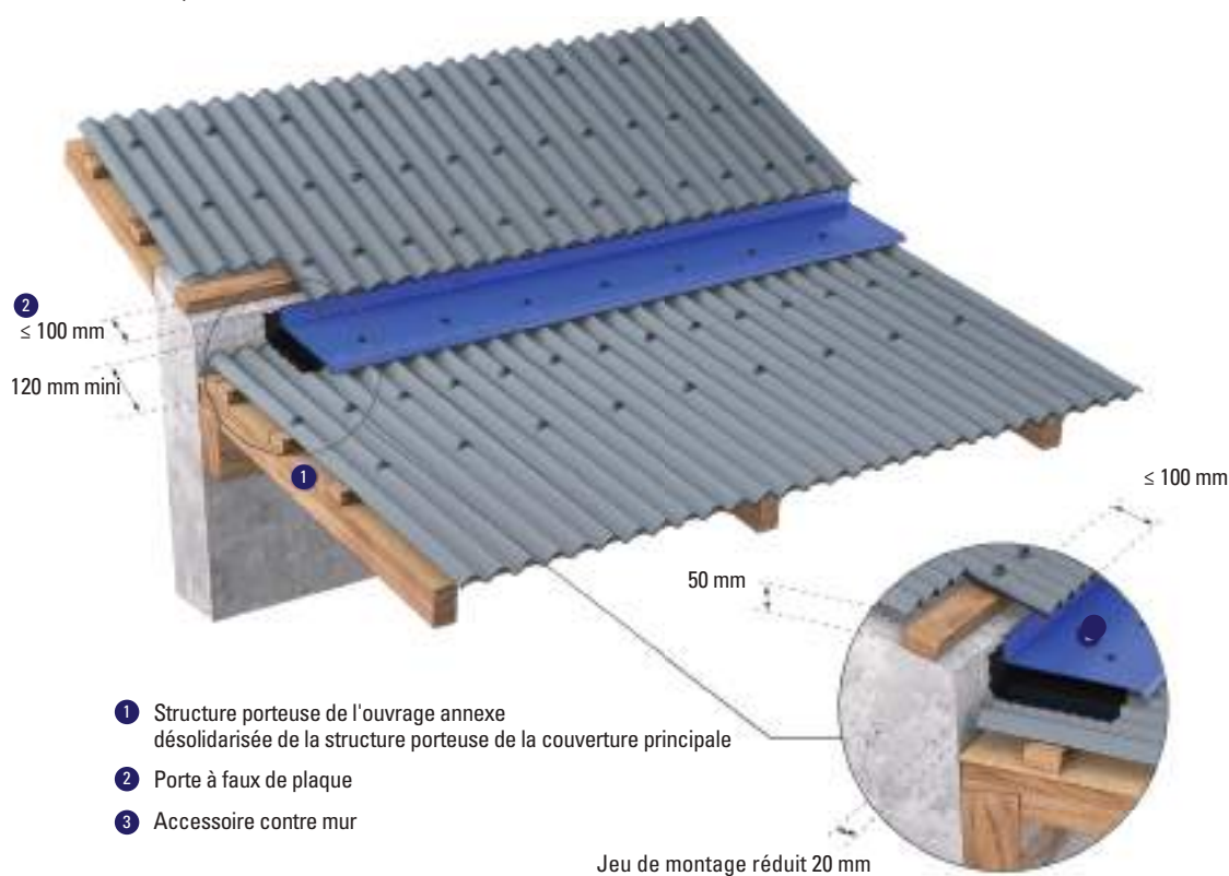
Figure 103 : Traitement avec ressaut de la jonction entre toiture principale et auvent
