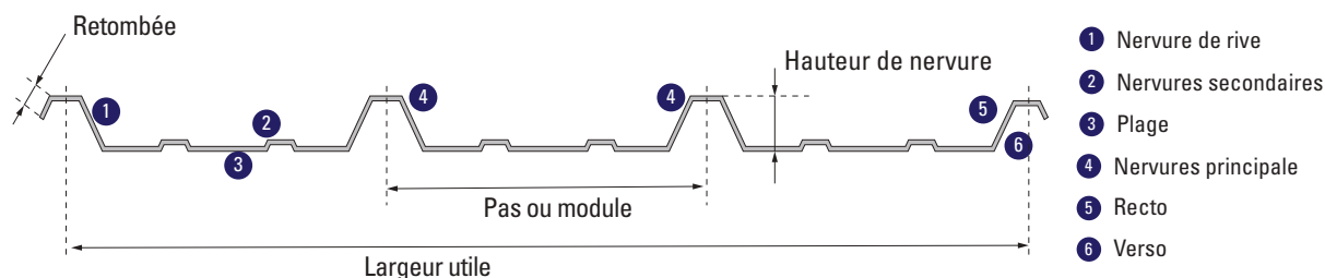
Figure 54 : Plaques nervurées – dénominations et paramètres
