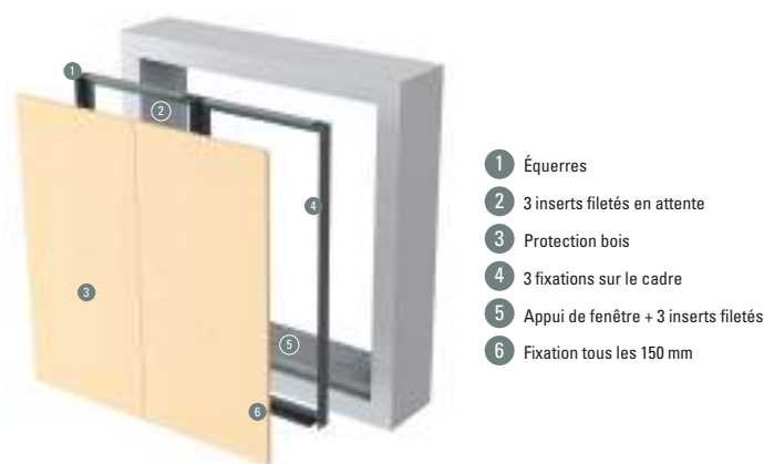
Figure 124 : Exemples de protection provisoire non poreuse (cas 3)
