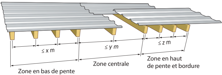
Figure 70 : Exemple d'une toiture à un versant - définition de trois zones
