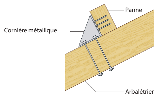
Figure 37 : Exemple de fixation des pannes sur l'arbalétrier par des cornières métalliques
