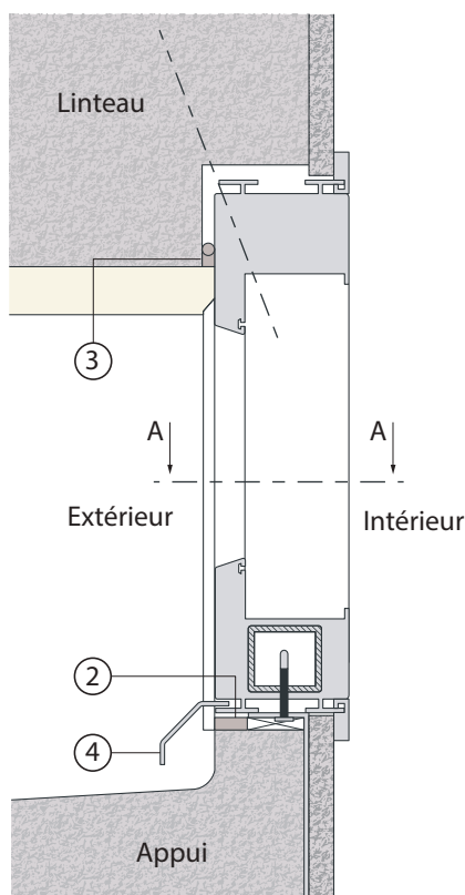
Figure 149 : Mise en œuvre en feuillure – Feuillure sèche maçonnerie niveau 1
