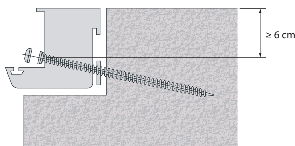
Figure 146 : Exemple de fixation par « vis à béton »
