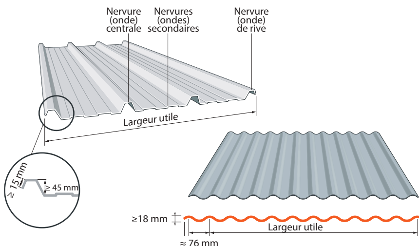
Figure 58 : Hauteur minimale des nervures
