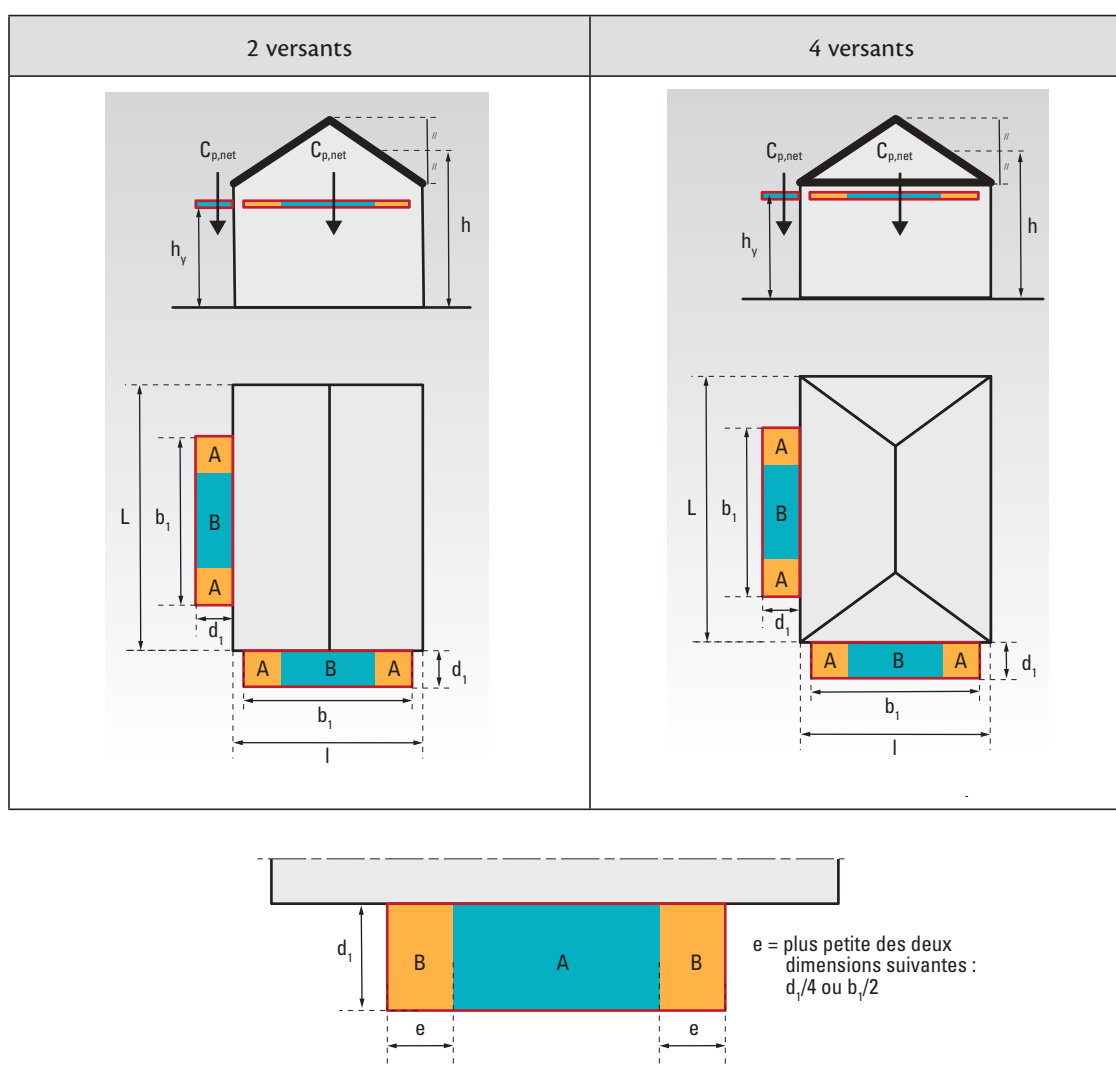
Figure 113 : Définition des zones de toiture selon le nombre de versants
