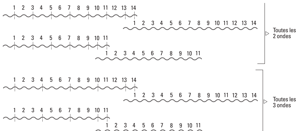
Figure 80 : Implantation des fixations aux recouvrements sur une couverture en tôles ondulées de 14 et 11 ondes
