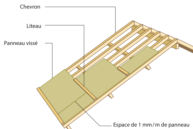
Figure 15 : Exemple de contreventement de versants par des plaques à base de bois
