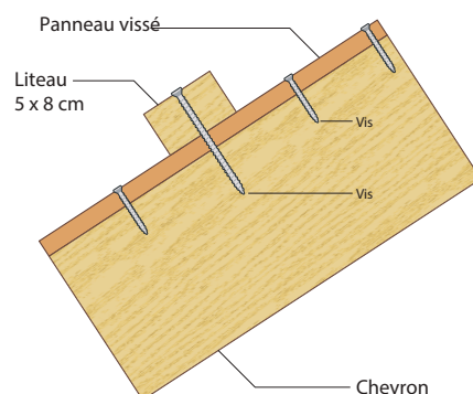
Figure 16 : Exemple de fixation de liteau sur le chevron au travers de la plaque
