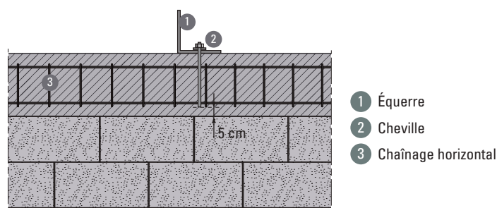
Figure 42 : Exemple de fixation dans un chaînage horizontal
