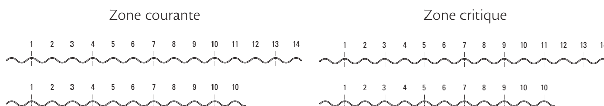
Figure 79 : Implantation des fixations sur une couverture en tôles ondulées de 14 et 11 ondes
