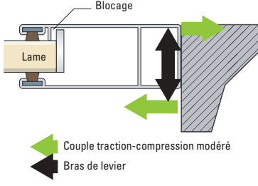
Figure 139 : Coulisse disposant d'un retour en tableau Disposition favorable
