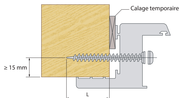
Figure 145 : Vissage direct dans le montant en bois existant
