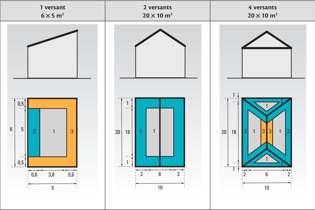
Figure 50 : Exemples de dimensions des zones de toiture selon le nombre de versants
