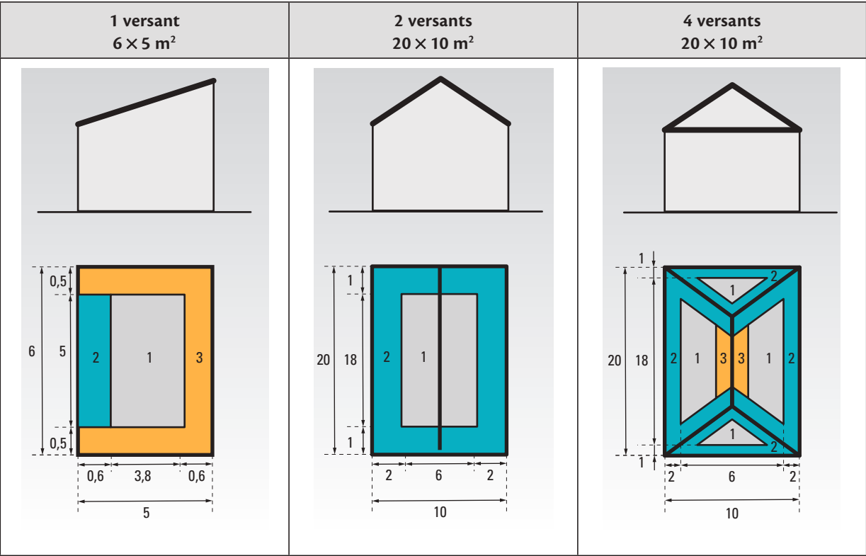
Figure 69 : Exemples de dimensions des zones de toiture selon le nombre de versants
