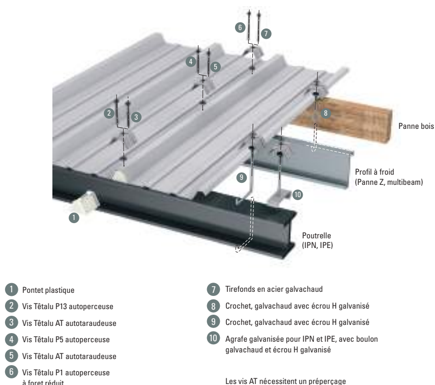
Figure 158 : Exemple de fixations sur toiture en tôle d'acier nervurée
