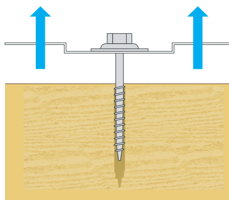
Figure 66 : Arrachement ou rupture d'une fixation
