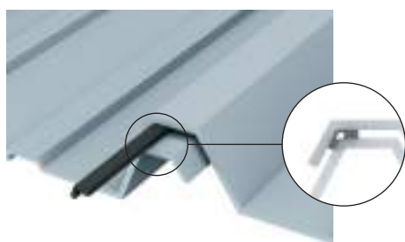
Figure 97 : Bande d'étanchéité
