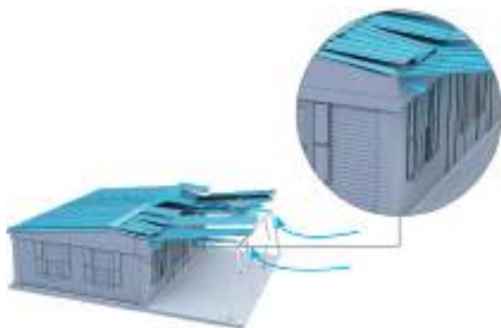
Figure 101 : Cas d'un auvent non désolidarisé
