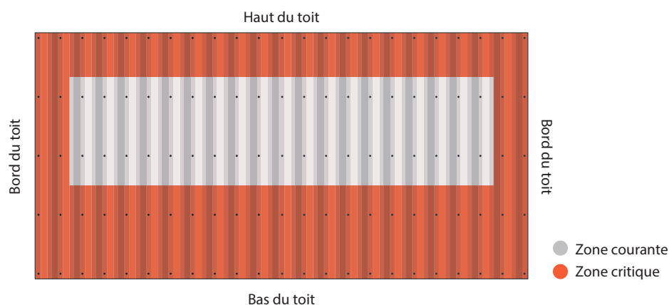
Figure 82 : Exemples de zones où disposer les pontets pour une toiture à un ou deux versants
