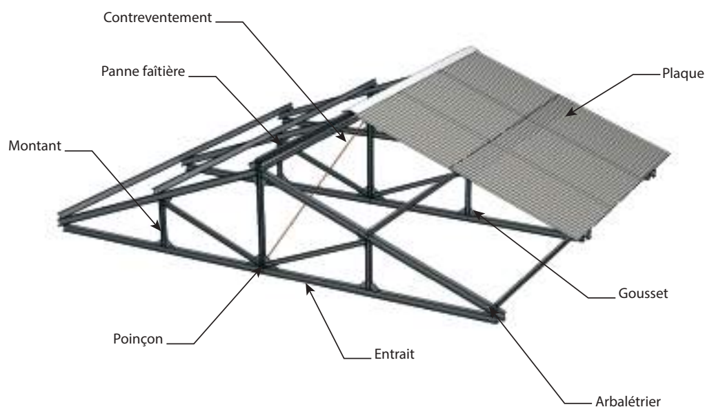
Figure 43 : Exemple de pannes sur arbalétrier
