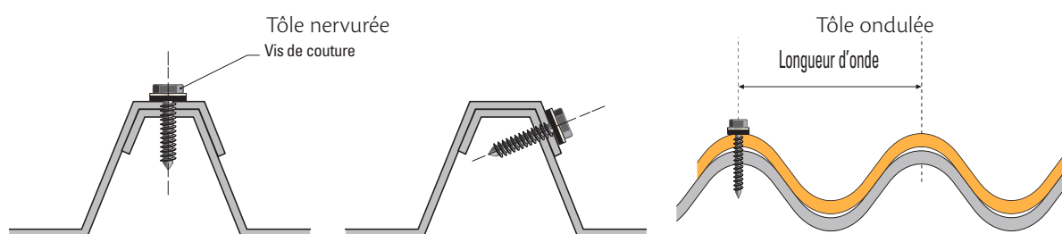
Figure 81 : Localisation des fixations de couture
