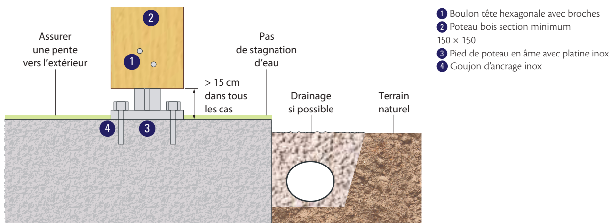
Figure 120 : Exemple de fixation au sol du pied de poteau de l'auvent
