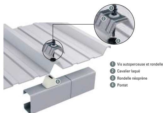
Figure 75 : Fixation d'une tôle nervurée avec pontet
