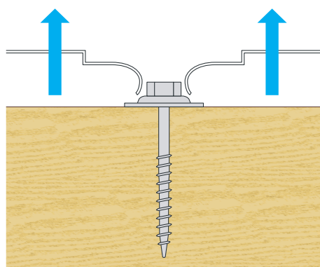
Figure 65 : Arrachement de la tôle au niveau d'une fixation
