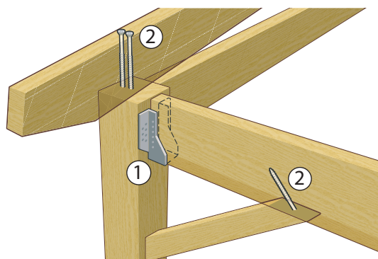
Figure 116 : Exemple d'équerre de fixation
