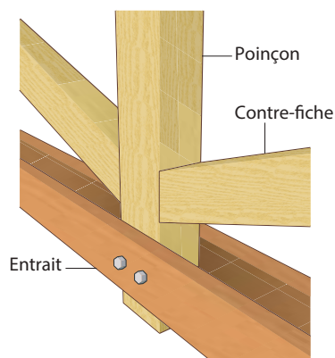
Figure 33 : Exemple d'assemblage entrain moisé - poinçon par 2 boulons
