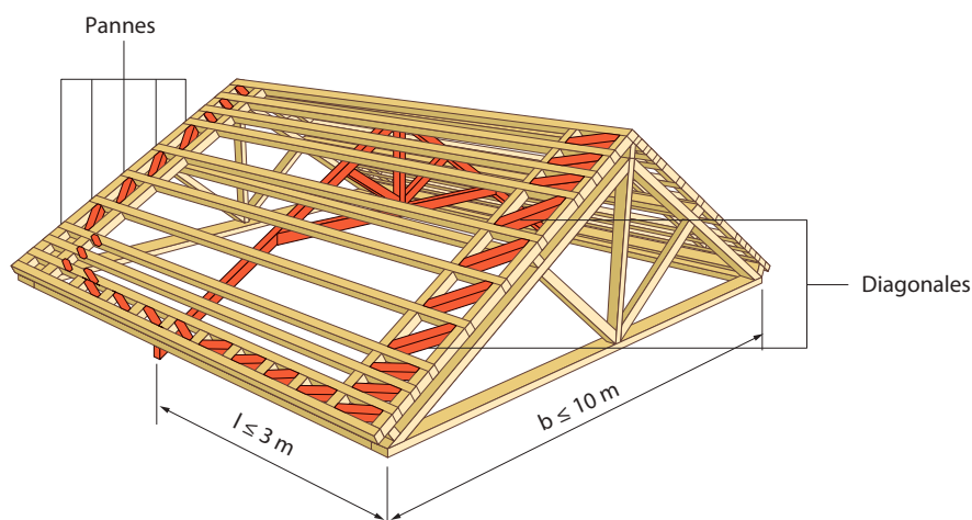
Figure 18 : Exemple de diagonales mises en œuvre entre pannes
