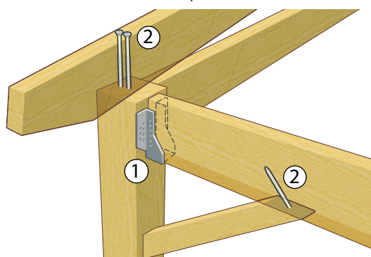
Figure 122 : Exemple de sabot à ailes extérieures inox
