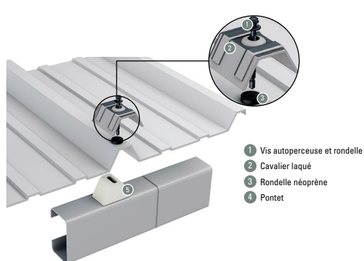
Figure 81 : Fixation d'une tôle nervurée avec pontet
