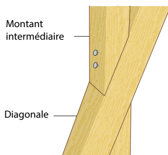
Figure 10 : Exemple de liaison diagonale – montant intermédiaire pour le cas d'une seule diagonale ou de deux diagonales non croisées
