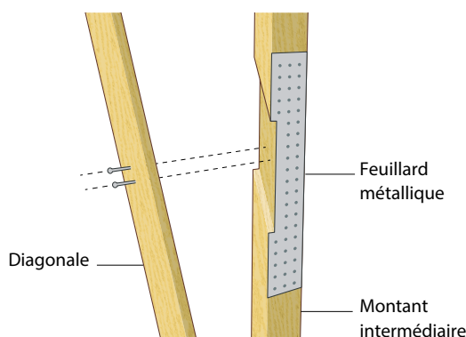
Figure 8 : Exemple de liaison diagonale – montant intermédiaire pour le cas de deux diagonales croisées
