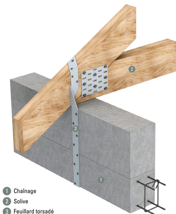
Figure 14 : Fixation des solives sur des chainages profonds
