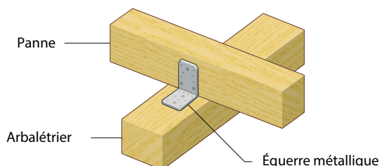
Figure 38 : Exemple de fixation des pannes sur l'arbalétrier par des équerres métalliques
