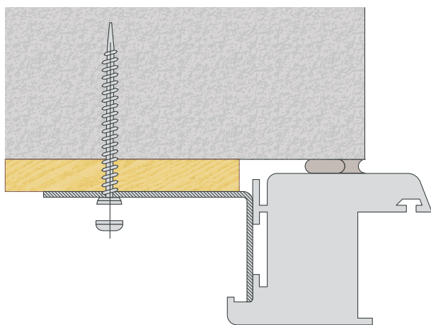
Figure 149 : Exemple de fixation par patte
