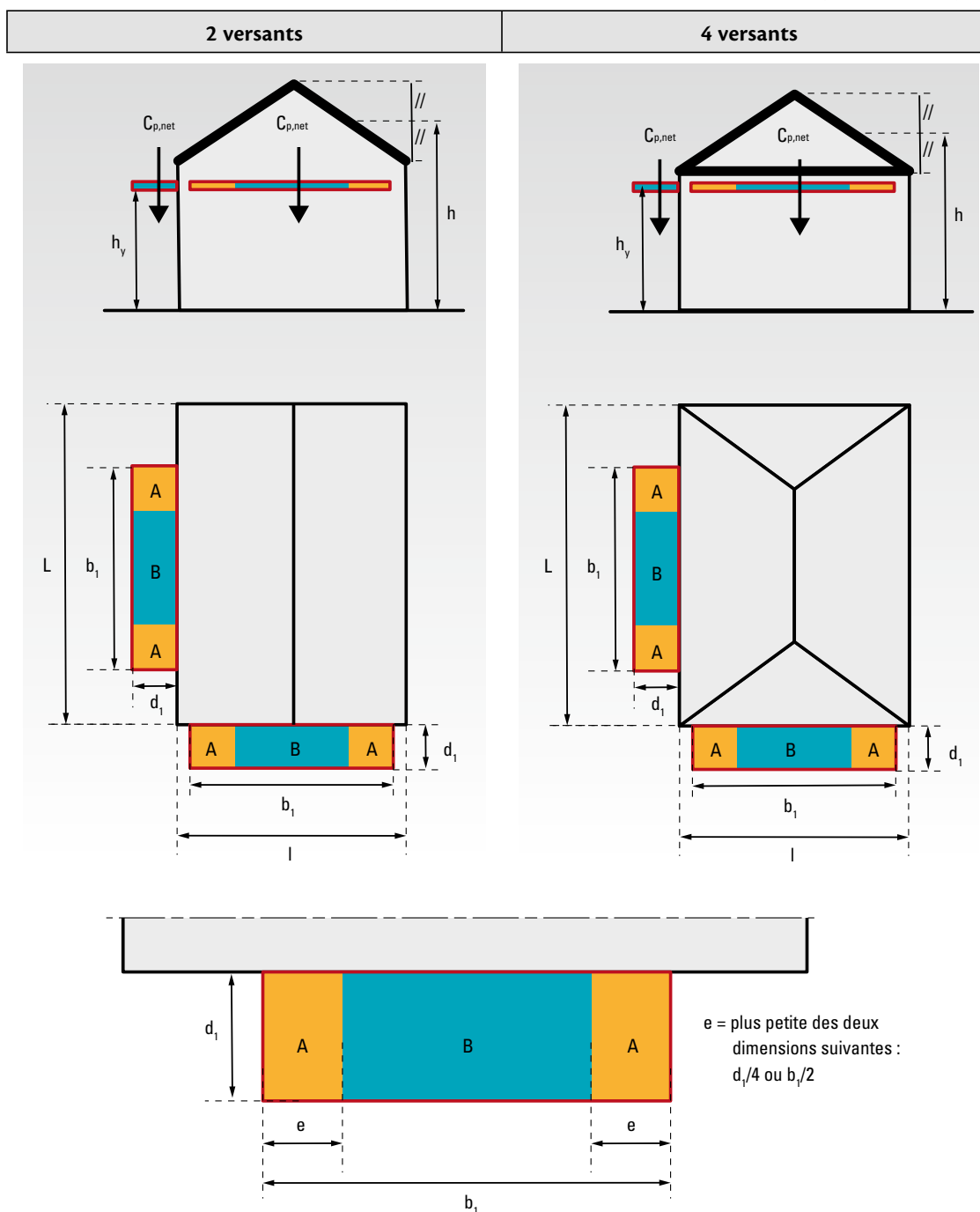
Figure 119 : Définition des zones de toiture selon le nombre de versants
