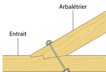
Figure 33 : Exemple d'assemblage entrain - arbalétrier par un boulon
