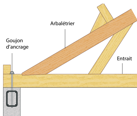
Figure 43 : Exemple d'ancrage de la charpente dans le béton par goujon d'ancrage
