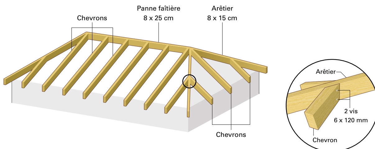
Figure 42 : Exemple de fixation des chevrons sur la panne faîtière par un boulon
