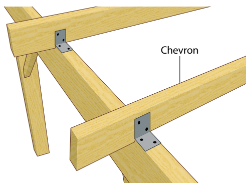
Figure 124 : Exemple d'équerre de fixation
