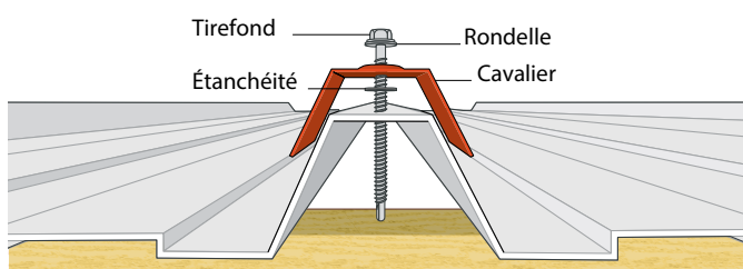
Figure 79 : Vue éclatée
