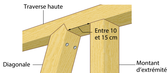
Figure 9 : Exemple de liaison diagonale – montant d'extrémité pour le cas d'une seule diagonale ou de deux diagonales non croisées
