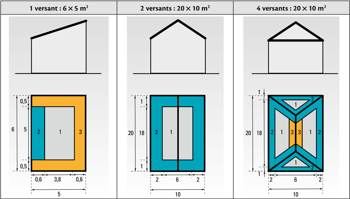
Figure 28 : Exemples de dimensions des zones de toiture selon le nombre de versants (projection sur le plan horizontal et non pas sur le plan des versants)
