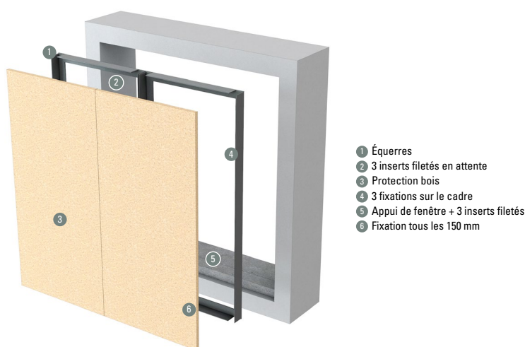
Figure 132 : Exemple d'un principe de protection provisoire
