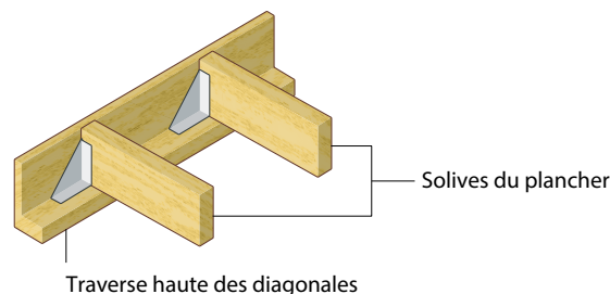
Figure 11 : Exemple de pose des solives sur la traverse haute du niveau bas
