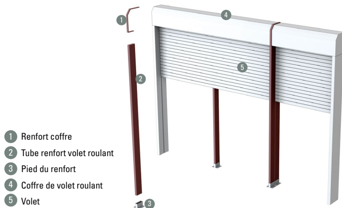
Figure 140 : Exemple de renforts sur volet roulant
