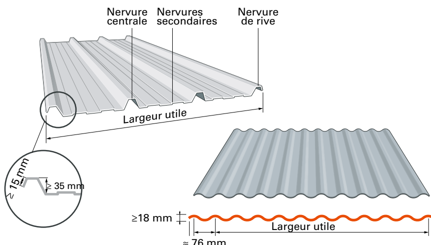
Figure 59 : Hauteur minimale des ondes (nervures)
