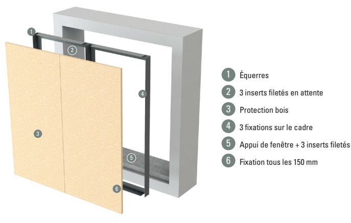
Figure 130 : Exemples de protection provisoire non poreuse (cas 3)
