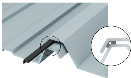
Figure 103 : Bande d'étanchéité
