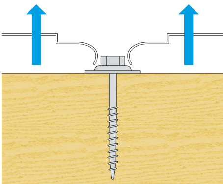
Figure 67 : Arrachement de la tôle au niveau d'une fixation
