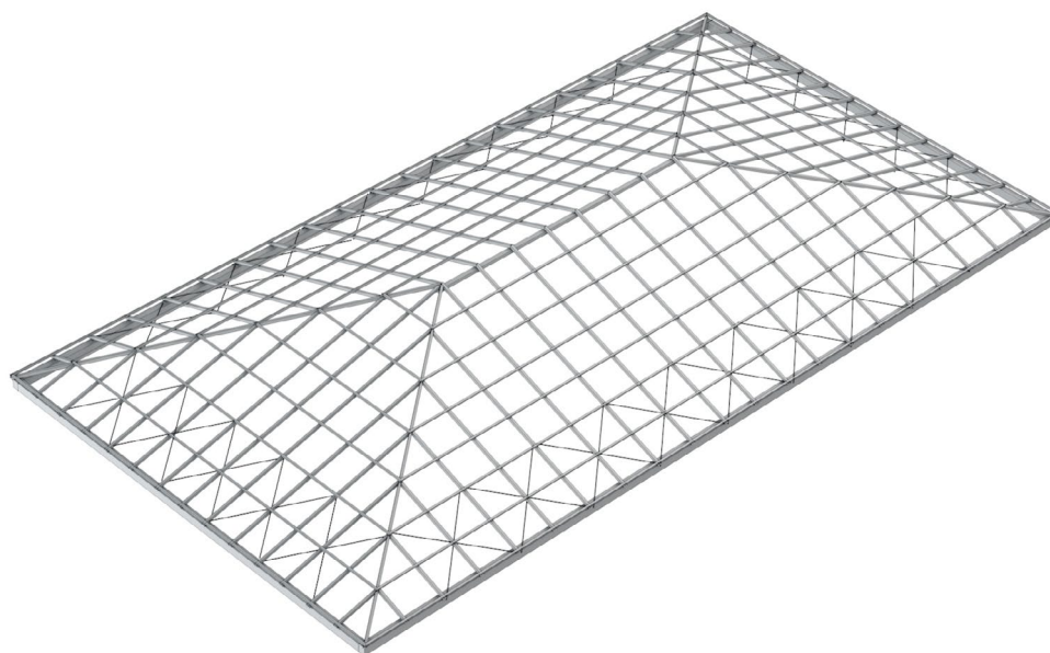
Figure 46 : Exemple d'une charpente à 4 versants
