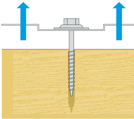
Figure 68 : Arrachement ou rupture d'une fixation
