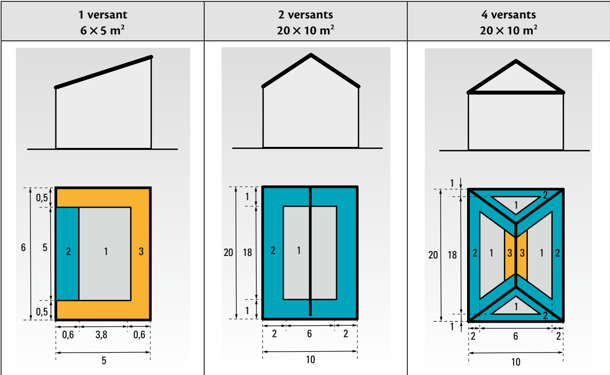
Figure 71 : Exemples de dimensions des zones de toiture selon le nombre de versants
