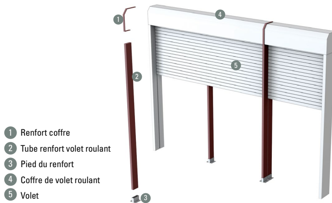
Figure 147 : Exemple de renforts sur volet roulant
