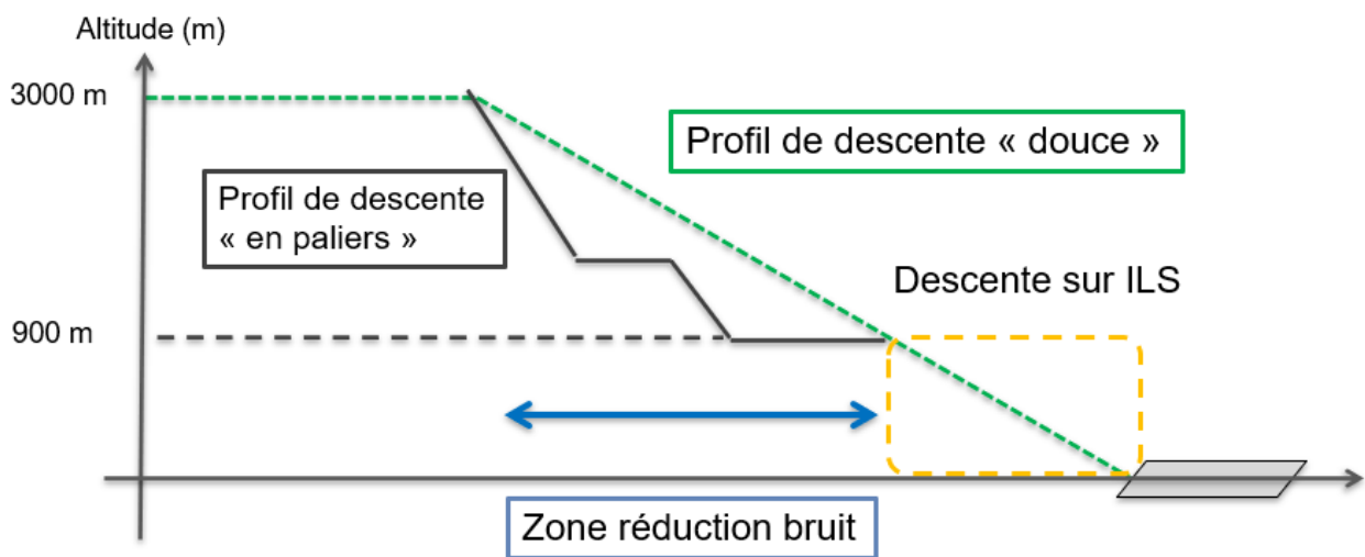
Figure 10 : Schéma d'un profil de descente continue ou descente douce
