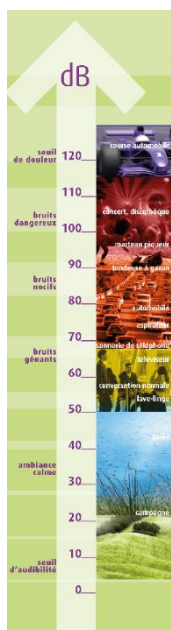
Figure 22 : Échelle des décibels (source : DGAC)
