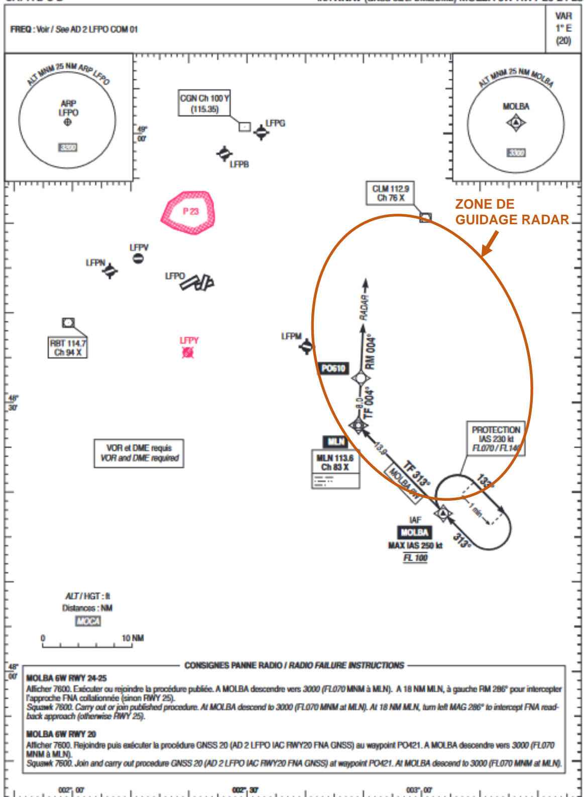
Figure 12 : Description schématique de la procédure RNAV (GNSS) MOLBA à LFPO pour la piste 3 QFU 25 (Carte 11P)
