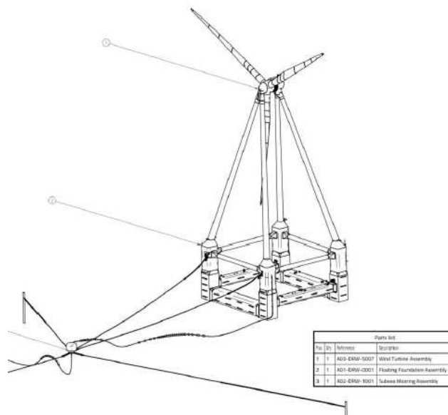
Démonstrateur 5 MW
